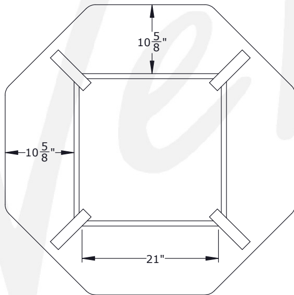
VUE DESSOUS / BOTTOM VIEW
