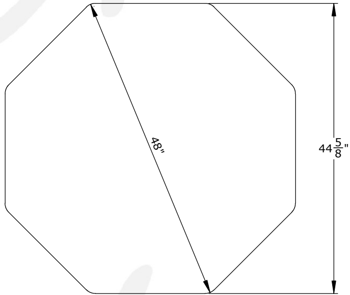
VUE DESSUS / TOP VIEW
